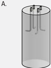
Poured Concrete L-bolts PART: L-Bolt-625
