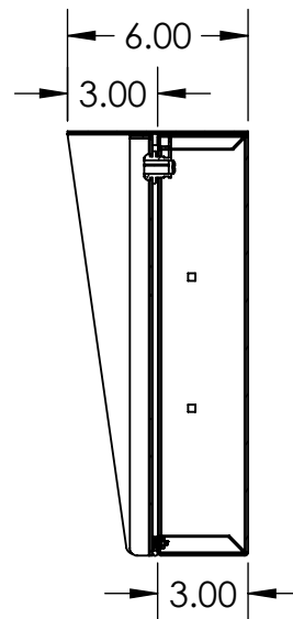
SECTION A-A
