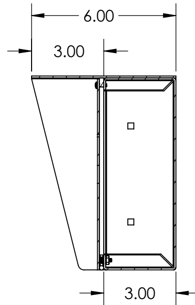
SECTION A-A
